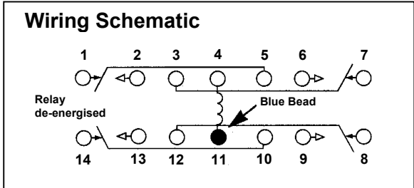
TYPE HDD4
