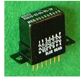
TYPE HDD4
